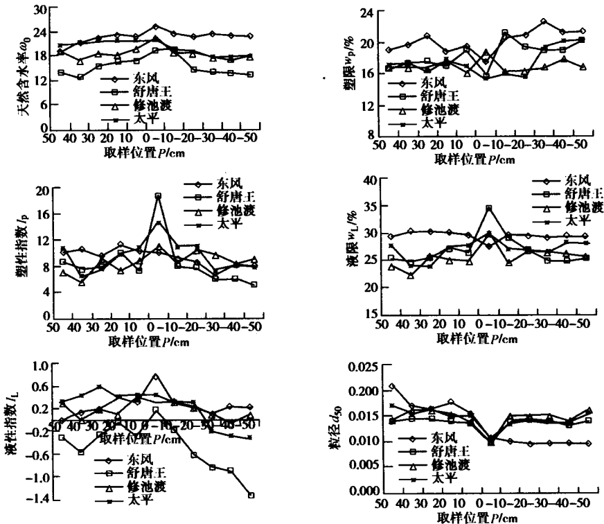
图 3 各物性指标与取样位置关系曲线
